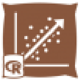
線形回帰
